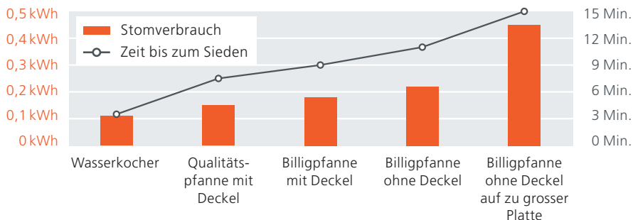
STROMVERBRAUCH UND ZEIT, UM 1 LITER WASSER ZUM SIEDEN ZU BRINGEN
