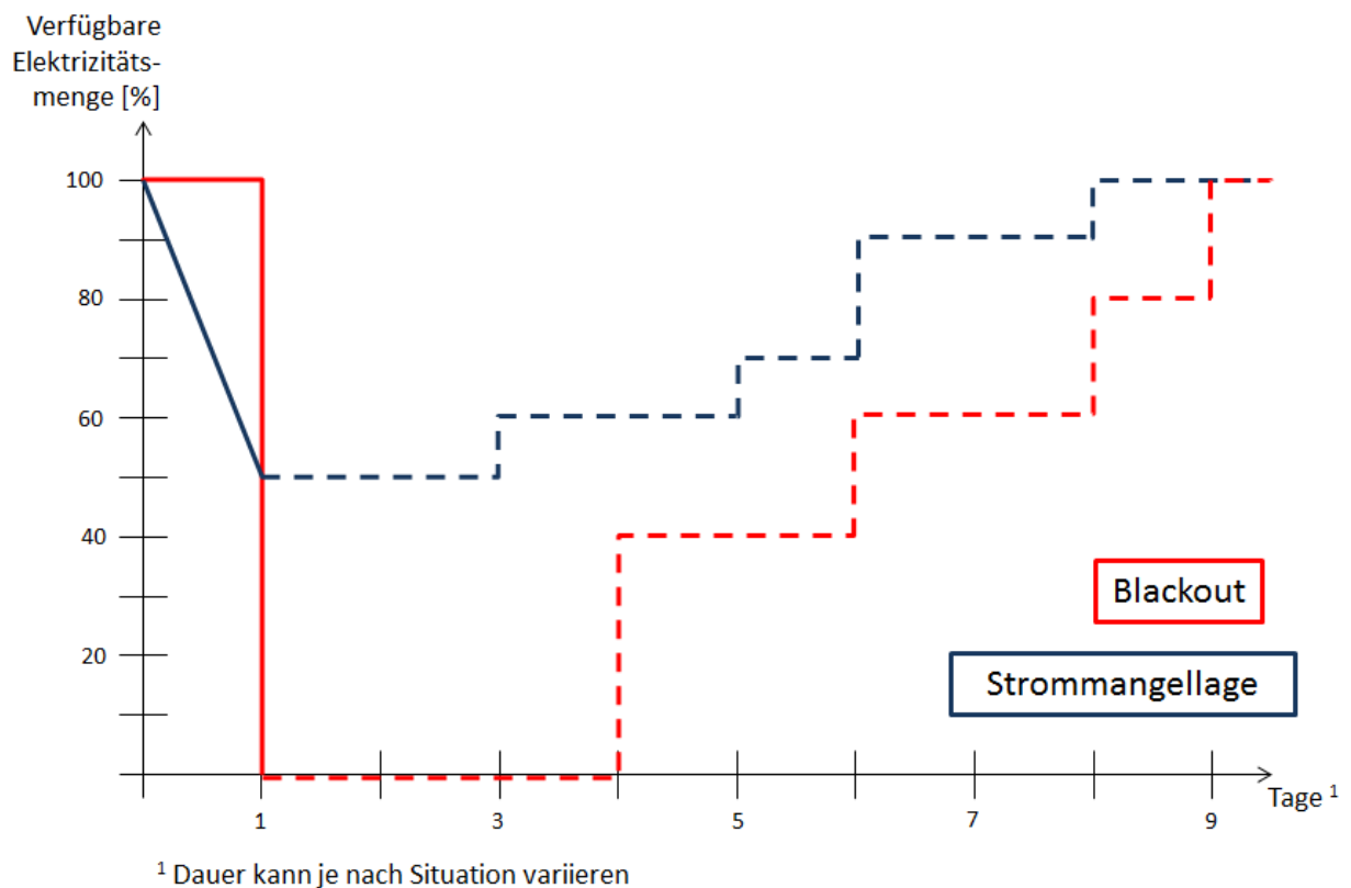
Abbildung 5: Schema (Neu-)Versorgung
