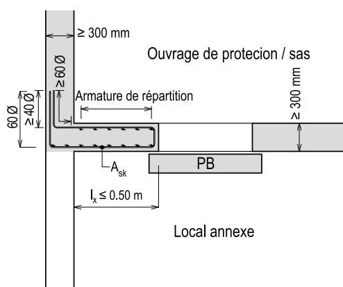
Figure 55 Tronçon de mur avec console
