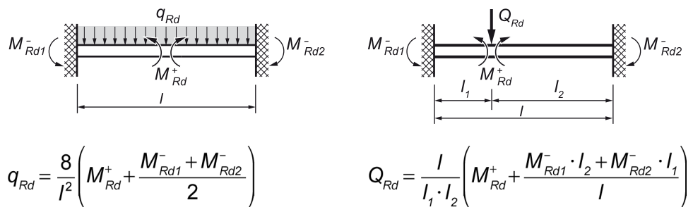
Figure 38 Charge ultime en flexion d'une poutre
