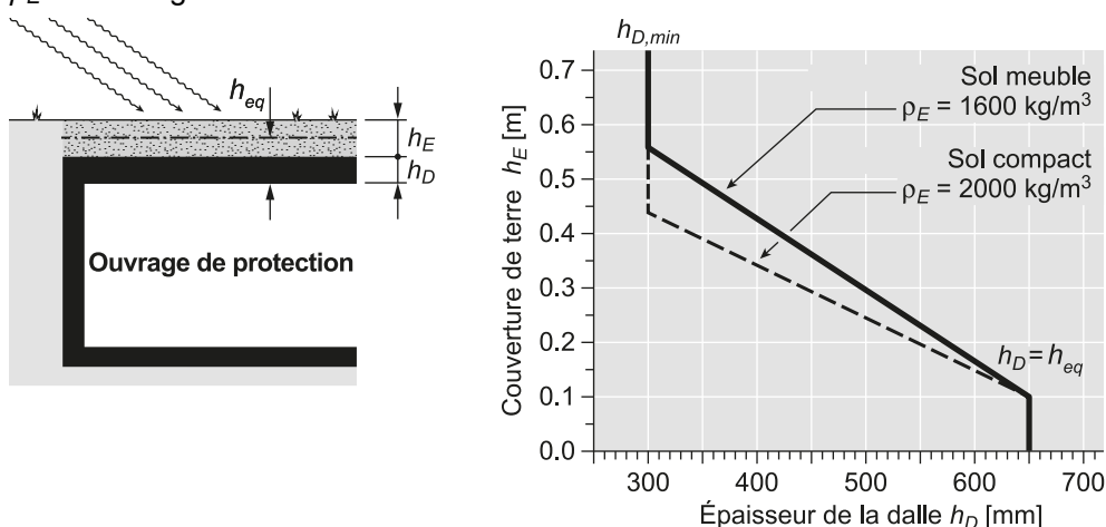
Figure 7 Épaisseur d'une dalle recouverte de terre
