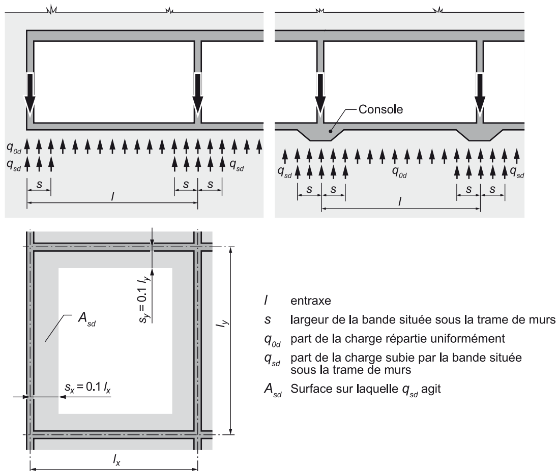
Figure 20 Actions sur le radier en présence d'une trame de murs
