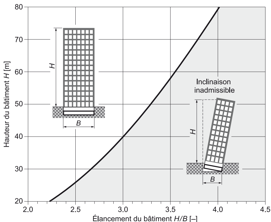
Figure 2 Risque d'atteindre une inclinaison inadmissible en fonction de la hauteur H et de l'élancement H/B du bâtiment
