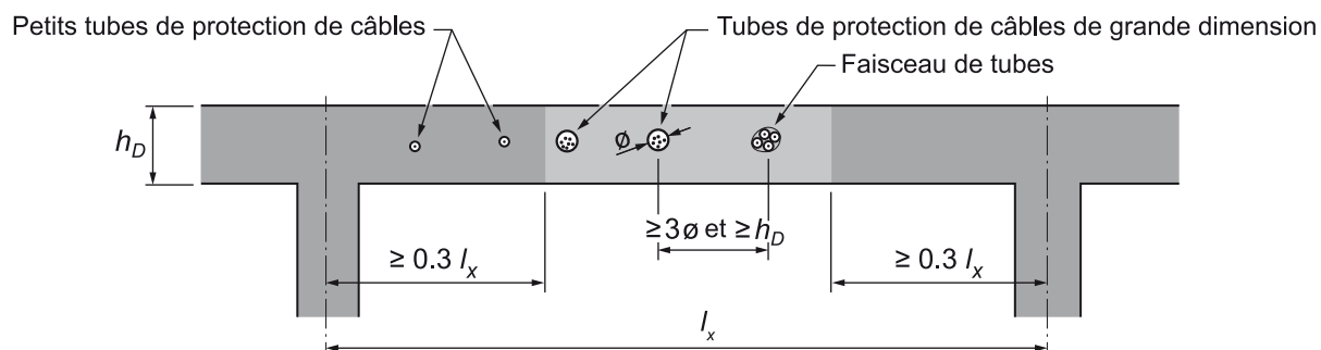
Figure 49 Conduites électriques et câbles de transmission placés dans des tubes de protection
