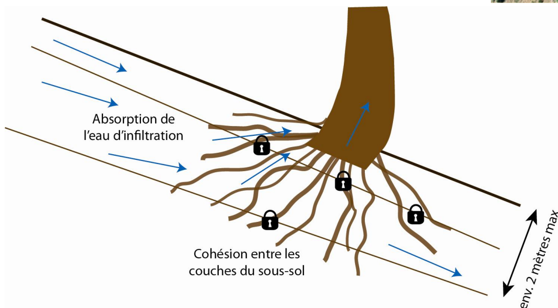
Figure 5 : Illustration des deux effets directs principaux de la forêt sur les glissements superficiels.
