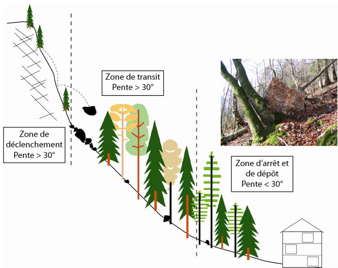
Figure 4 : Illustration des trois zones d'influences de la forêt contre les chutes de pierres.
