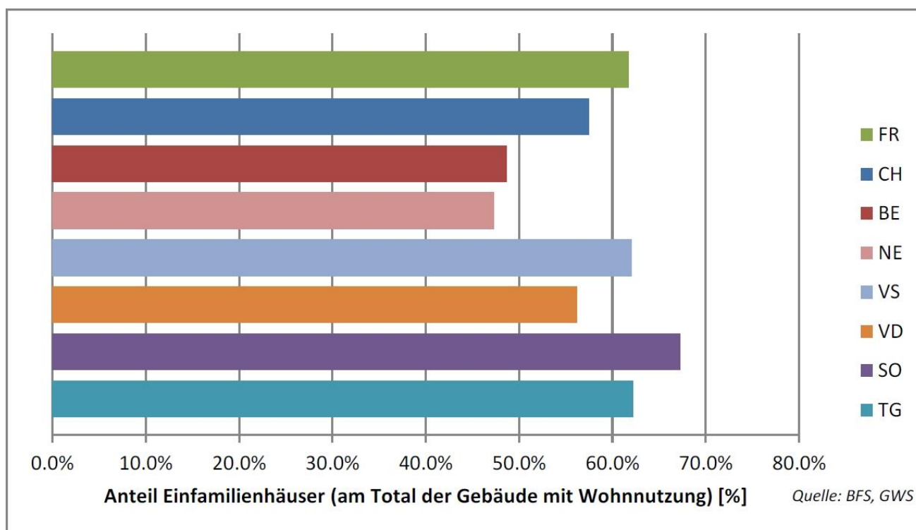
Abbildung 8: Anteil Einfamilienhäuser
