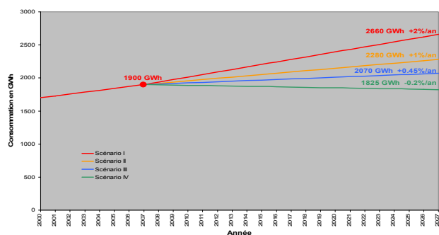
Evolution de la consommation d'électricité en fonction des scénarios I, II, III, et IV des perspectives énergétiques de la Confédération adaptées au canton de Fribourg
